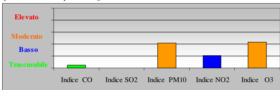
Fig.2 Giudizi di qualità dell'aria – stazioni Luglio 2012
