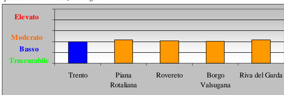
Fig.2 Giudizi di qualità dell'aria – stazioni Luglio 2012
