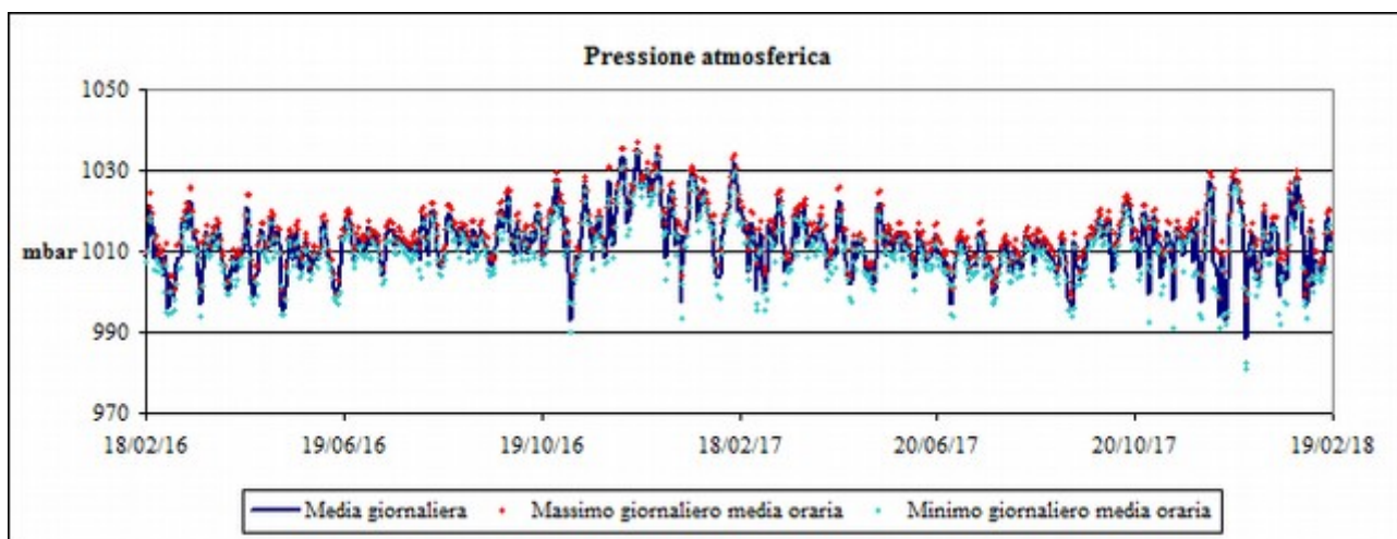
Fig. 3.9: Pressione atmosferica.
