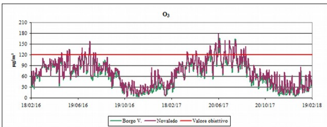
Fig. 4.22: O 3 – Massimo giornaliero media 8 h (Novaledo e Borgo Valsugana).
