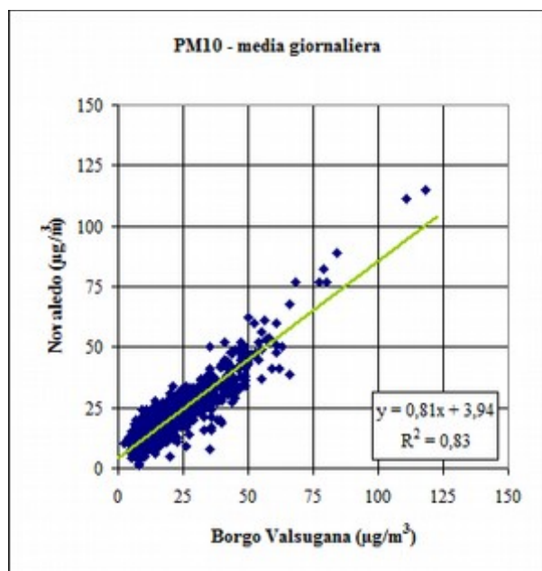
Fig. 4.8: PM10 – Retta di correlazione (Novaledo – Borgo Valsugana).
