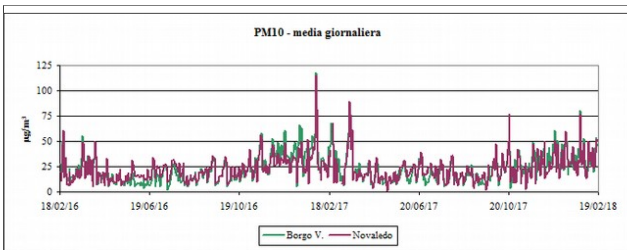
Fig. 4.5: PM10 – Media giornaliera (Novaledo e Borgo Valsugana).
