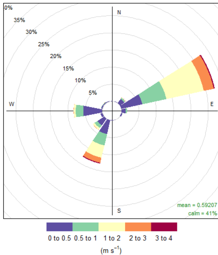
Fig. 3.3: Rosa dei venti.
