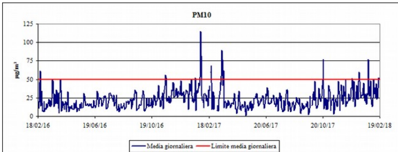
Fig. 4.4: PM10 – Media giornaliera.
