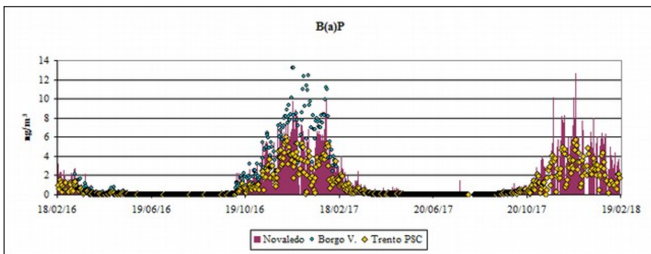
Fig. 4.27: B(a)P – Media giornaliera (Novaledo, Trento Parco S. Chiara e Borgo Valsugana).
