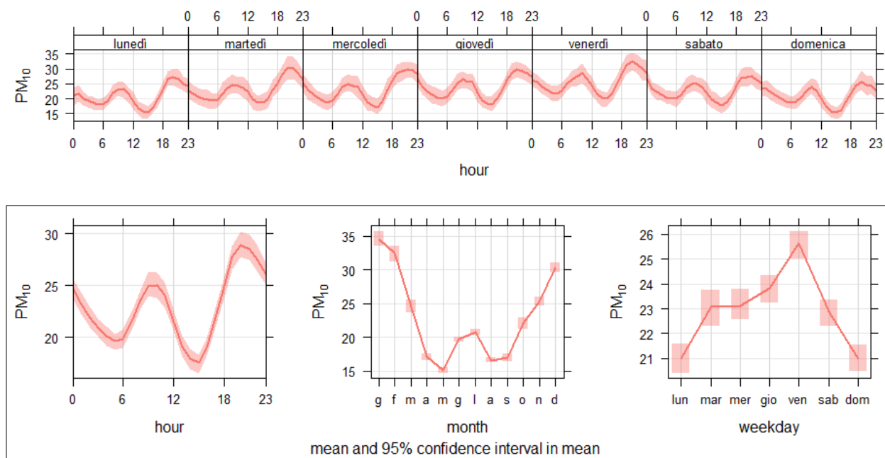
Fig. 4.7: Andamenti PM10 ( \mu\text{g}/\text{m}^3 ).
