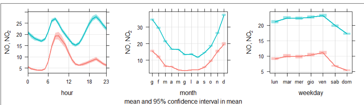
Fig. 4.18 NO ed NO 2 – Andamenti (valori normalizzati).
