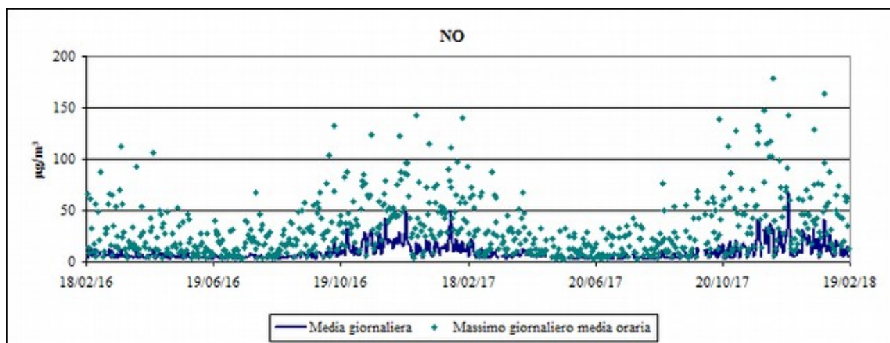
Fig. 4.10: NO – Media giornaliera e massimo orario.
