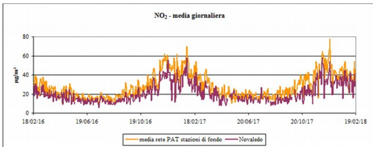
Fig. 4.13: NO 2 – Media giornaliera (Novaledo e media rete PAT).
