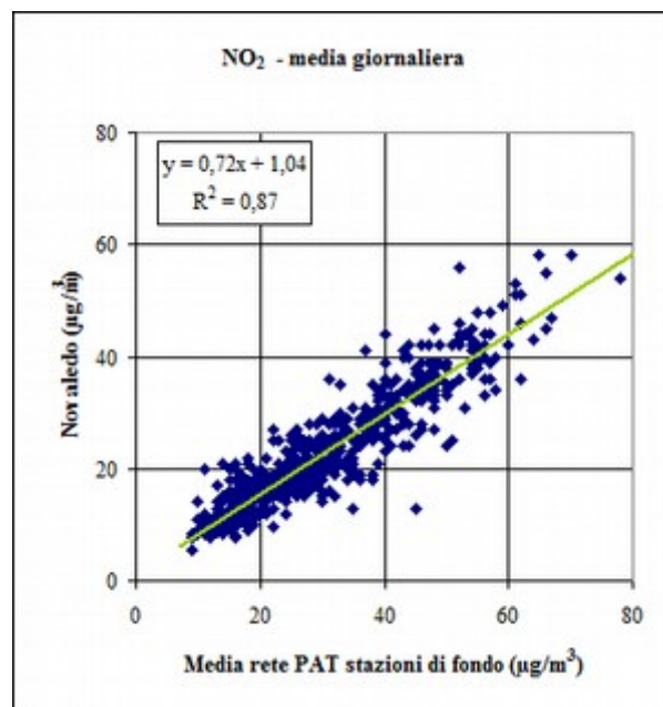
Fig. 4.15: NO 2 – Retta di correlazione (Novaledo – media rete PAT stazioni di fondo).
