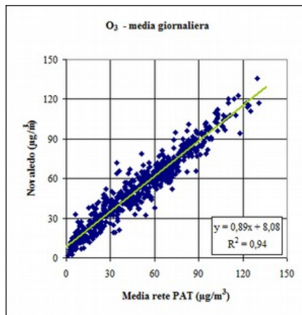
Fig. 4.24: O 3 – Retta di correlazione (Noaledo – media rete PAT).
