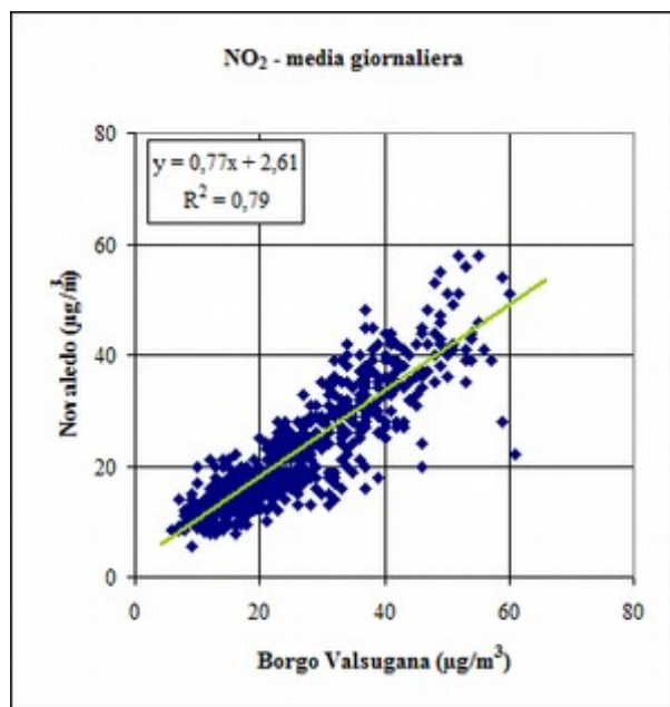
Fig. 4.14: NO 2 – Retta di correlazione (Novaledo – Borgo Valsugana).
