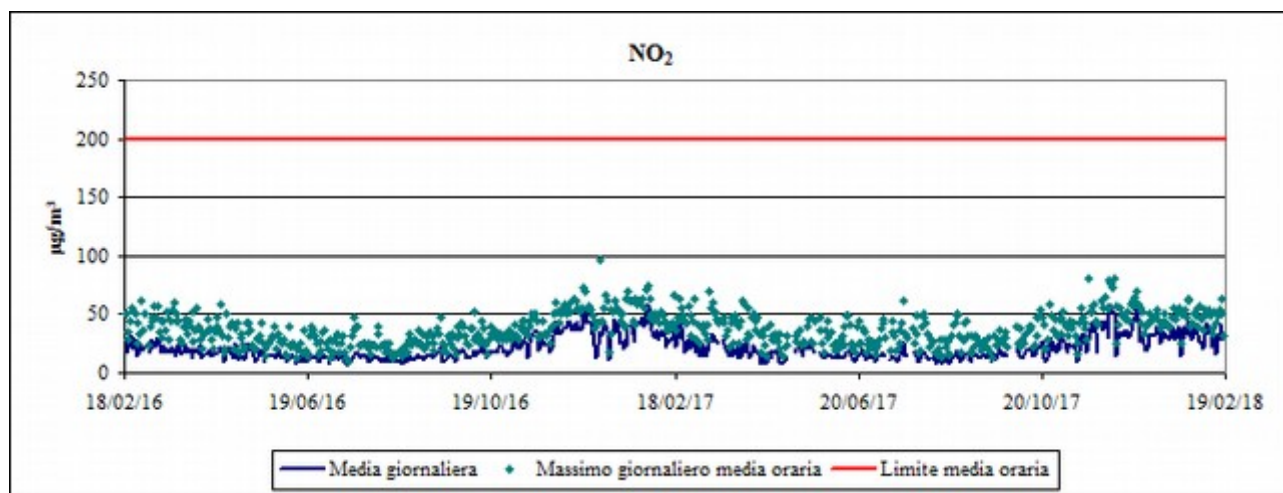
Fig. 4.11: NO 2 – Media giornaliera e massimo orario.
