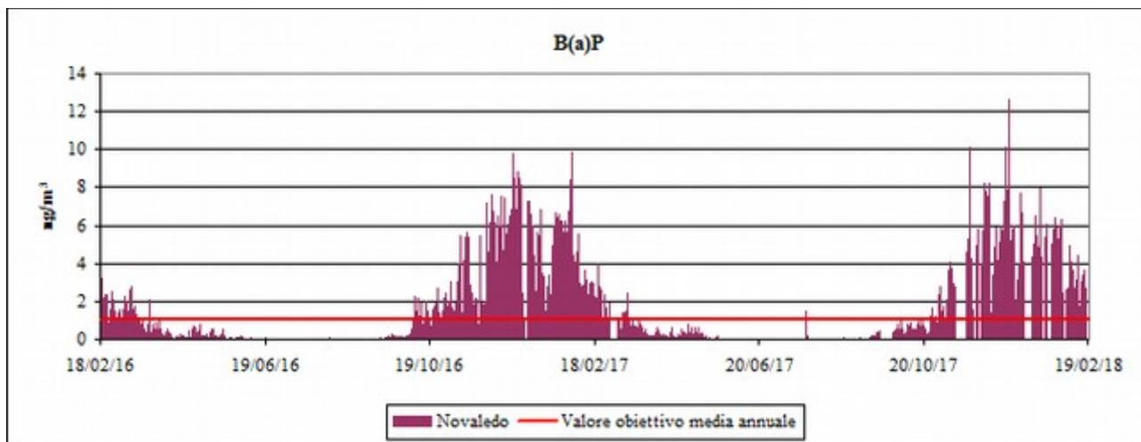
Fig. 4.26: B(a)P – Media giornaliera.
