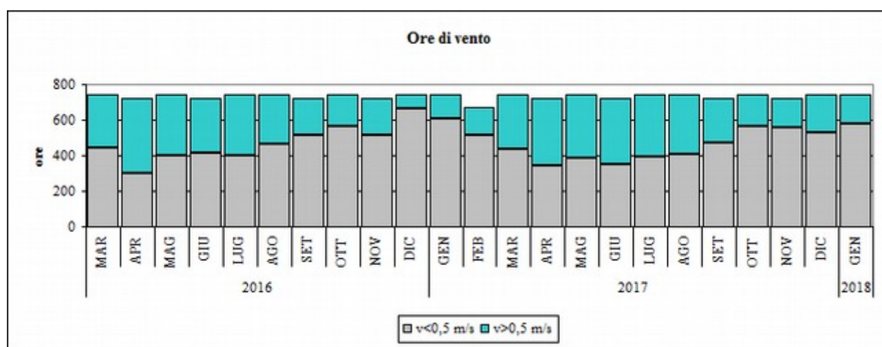
Fig. 3.2: Ore di vento mensili (velocità maggiore e minore di 0,5 m/s).
