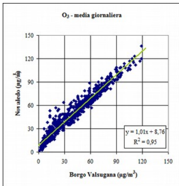
Fig. 4.23: O 3 – Retta di correlazione (Noaledo – Borgo Valsugana).
