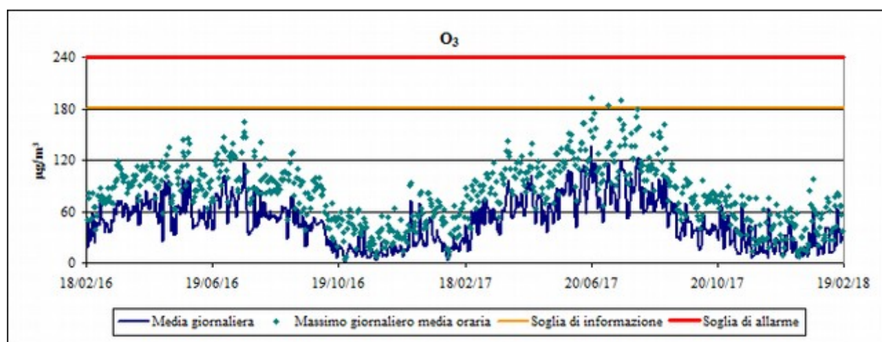
Fig. 4.19: O 3 – Media giornaliera e massimo orario.
