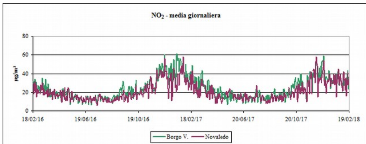
Fig. 4.12: NO 2 – Media giornaliera (Novaledo e Borgo Valsugana).
