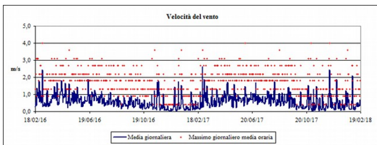
Fig. 3.1: Velocità del vento.
