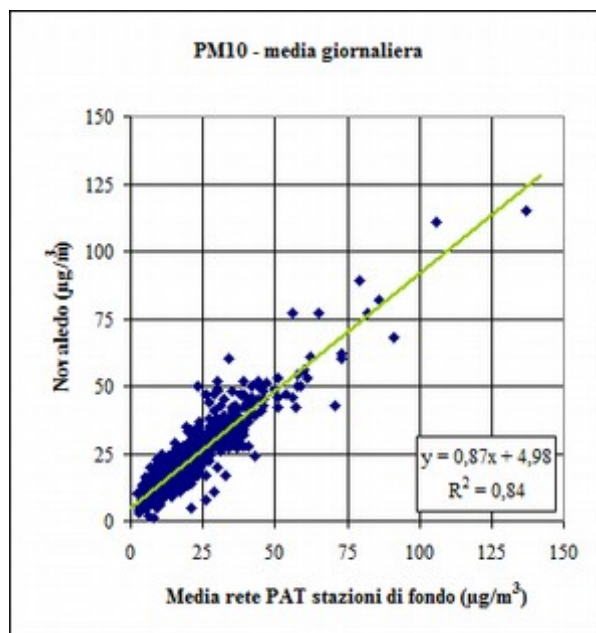
Fig. 4.9: PM10 – Retta di correlazione (Novaledo - media rete PAT stazioni di fondo).
