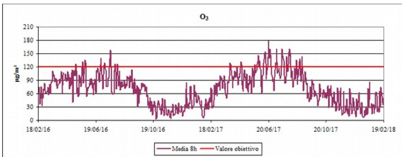
Fig. 4.21: O 3 – Massimo giornaliero media 8 h.
