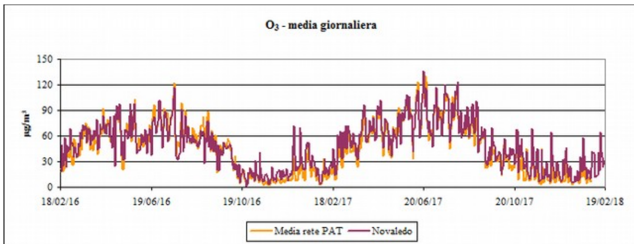
Fig. 4.20: O 3 – Media giornaliera (Novaledo e media rete PAT).
