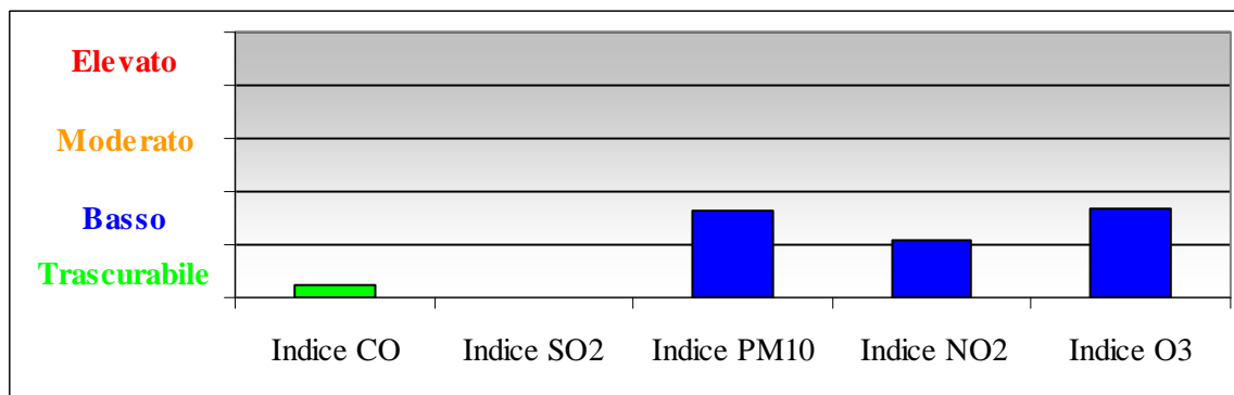
Fig.2 Giudizi di qualità dell'aria – stazioni – Aprile 2015
